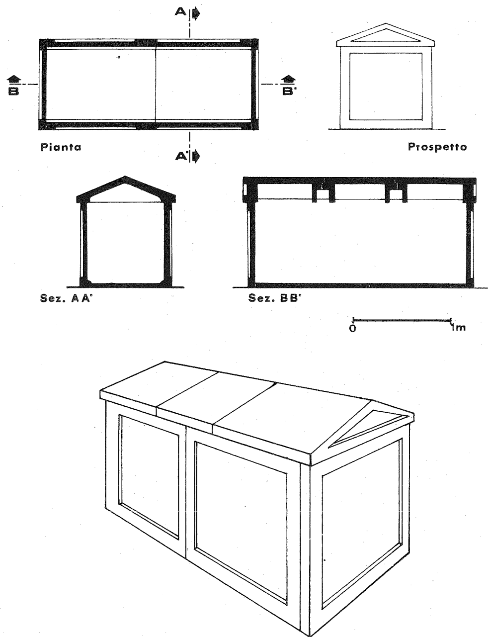
Fig. 5 - Pianta, prospetto, sezioni ed assonometria della tomba n. 16.
